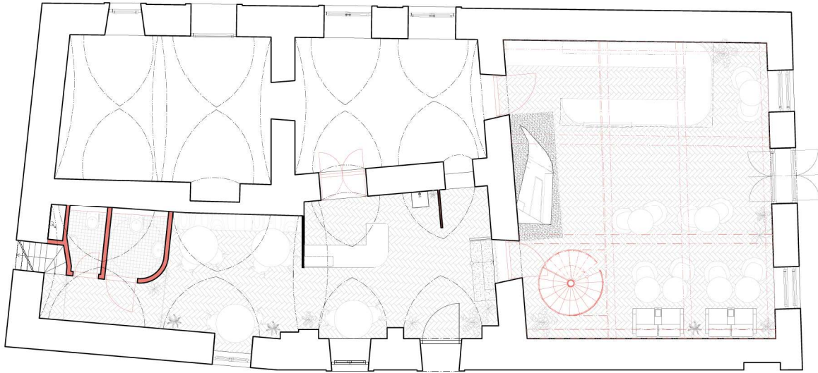
Pôdorys 1.NP
